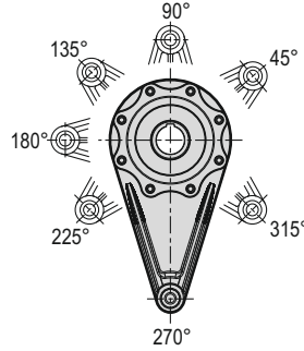
Tork kolunun pozisyonlanması Positions of torque arm / Positionierung der Drehmomentstütze
