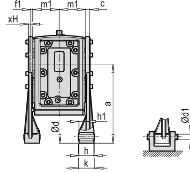
Tork kolunun pozisyonlanması Positions of torque arm / Positionierung der Drehmomentstütze
