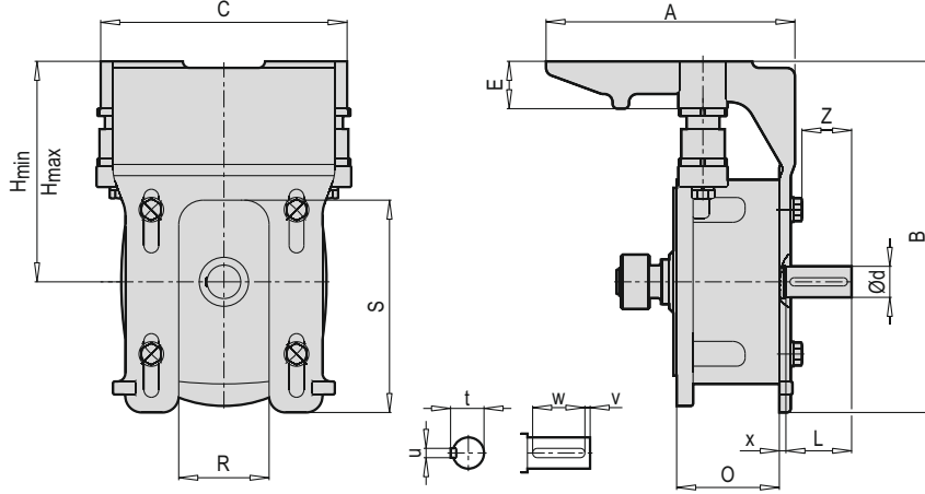
Motor Platformu Ölçüleri / Motor Platform Dimensions / Abmessungen der Motorkonsole
