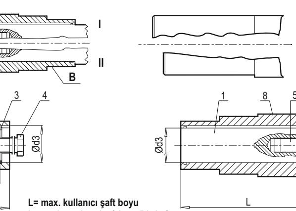
MONTAJ / ASSEMBLY
