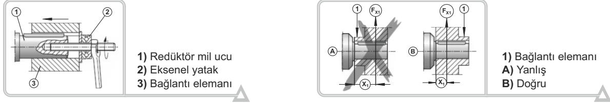
Şekil 6: Bağlantı Elemanının Çıkış Miline Montajı
