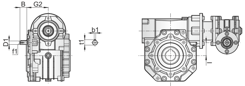
Şekil 16: Giriş Mili (ISV / SV)
