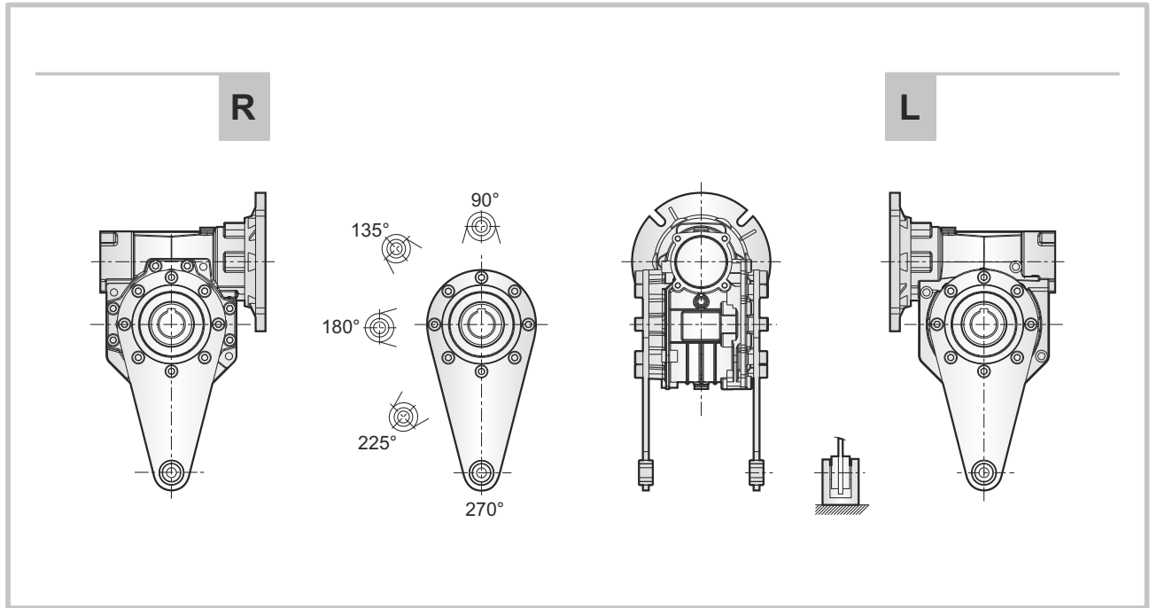
Şekil 14: Tork Kolu
