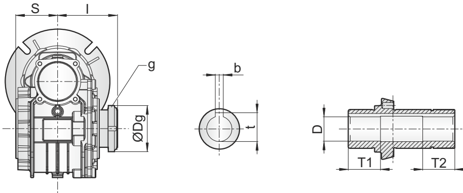
Şekil 19: Tork Sınırlayıcı
