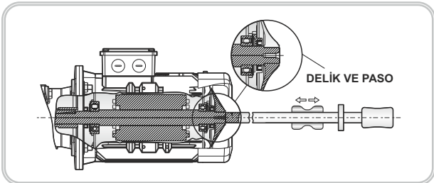
Şekil 8: Elektrik Motorunun Demontajı (PAM)
