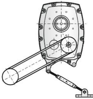
Şekil 14: V Kayışı ve Tork Kolu Bağlantısı (P)
