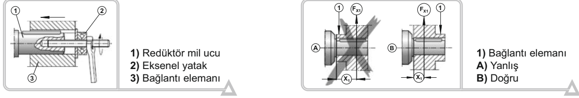
Şekil 7: Bağlantı Elemanının Çıkış Miline Montajı
