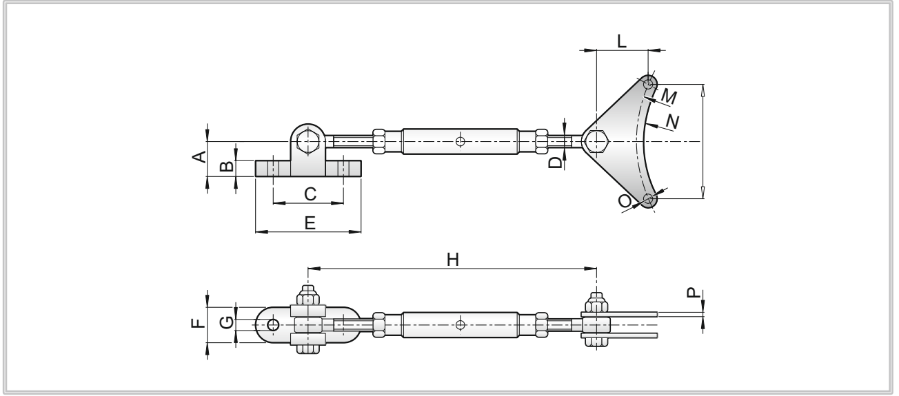
Şekil 21: Tork Kolu (Pt/A)
