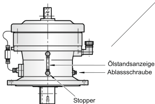
Abbildung 14: Öableitung bei vertikalen Typen
