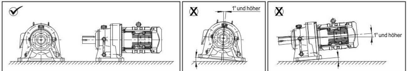
Abbildung 3: Montagewinkel (Beispielmontagetyp)
