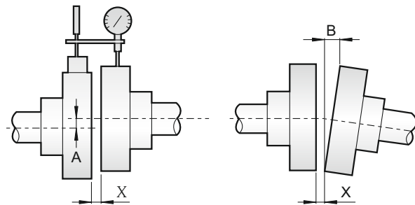
Abbildung 7-1: Ausrichtungsgenauigkeit
