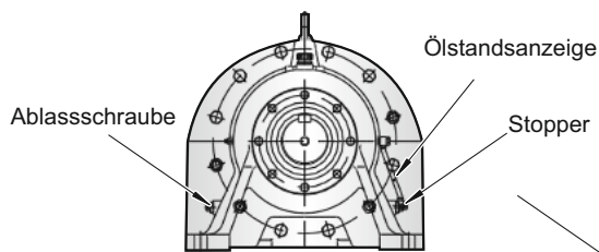
Abbildung 13: Öableitung bei horizontalen Ausführungen
