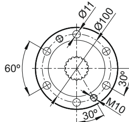
Trommelanschlussflanschmaße und - Toleranzen
