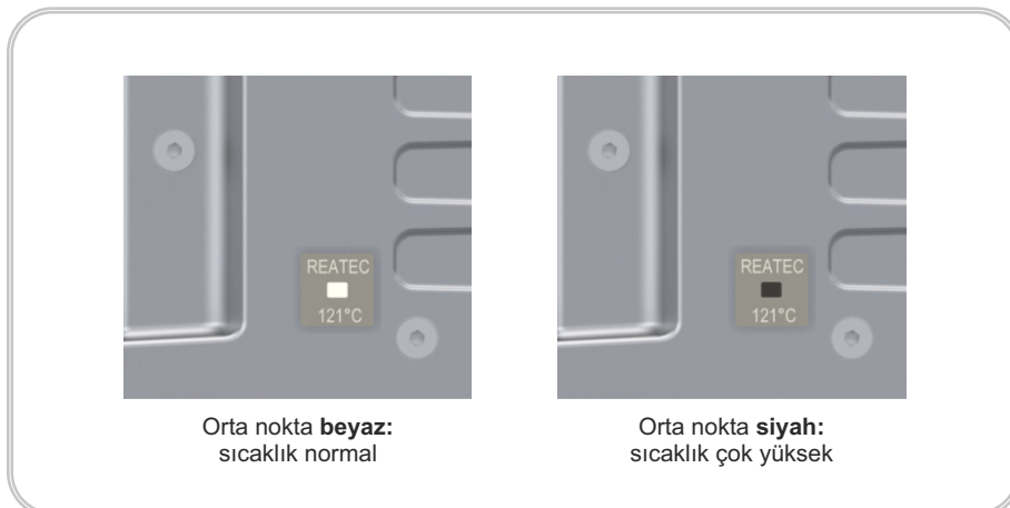
Şekil 11: Sıcaklık Etiketleri
