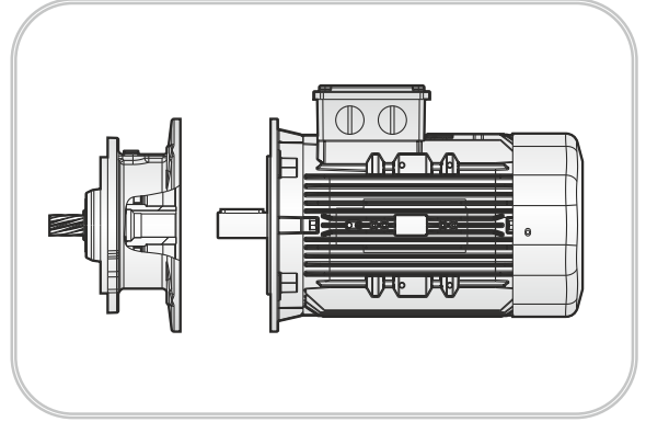
Şekil 8: Standart Bir B5 Motorunun PAM'lı Redüktöre Montajı
