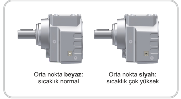
Şekil 5: Sıcaklık Etiketi (F)
