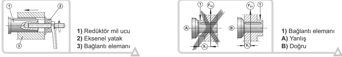
Şekil 6: Bağlantı Elemanının Çıkış Miline Montajı
