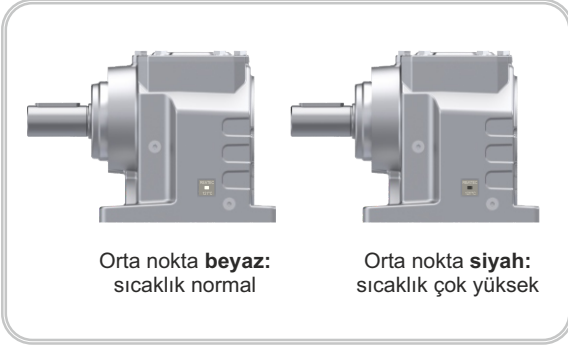
Şekil 4: Sıcaklık Etiketi (A / F)
