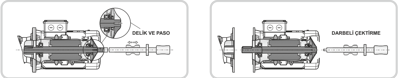
Şekil 9: Elektrik Motorunun Demontajı (PAM)
