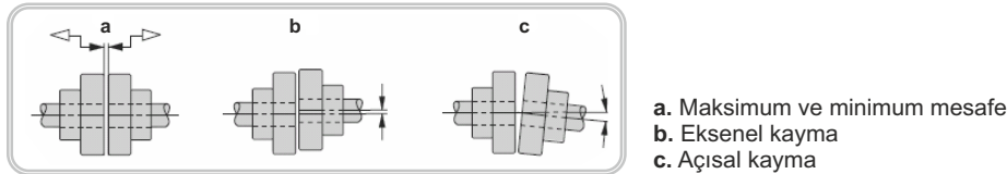
Şekil 7: Kaplin Montajı
