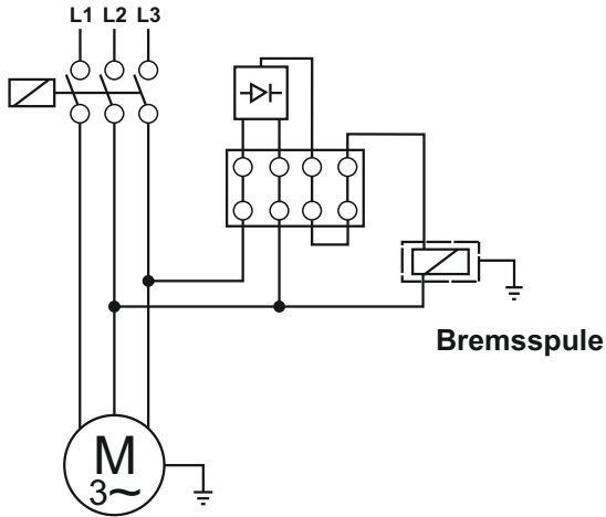
Abbildung 9: Standard Motorbremsen Anschlusschema
