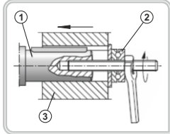
Şekil 4: Bağlantı Elemanının Çıkış Miline Montajı
