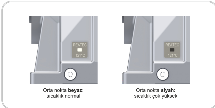
Şekil 9: Sıcaklık Etiketleri 2
