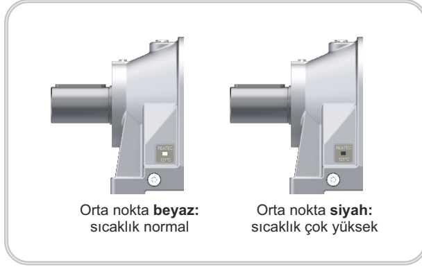
Şekil 5: Sıcaklık Etiketi 1
