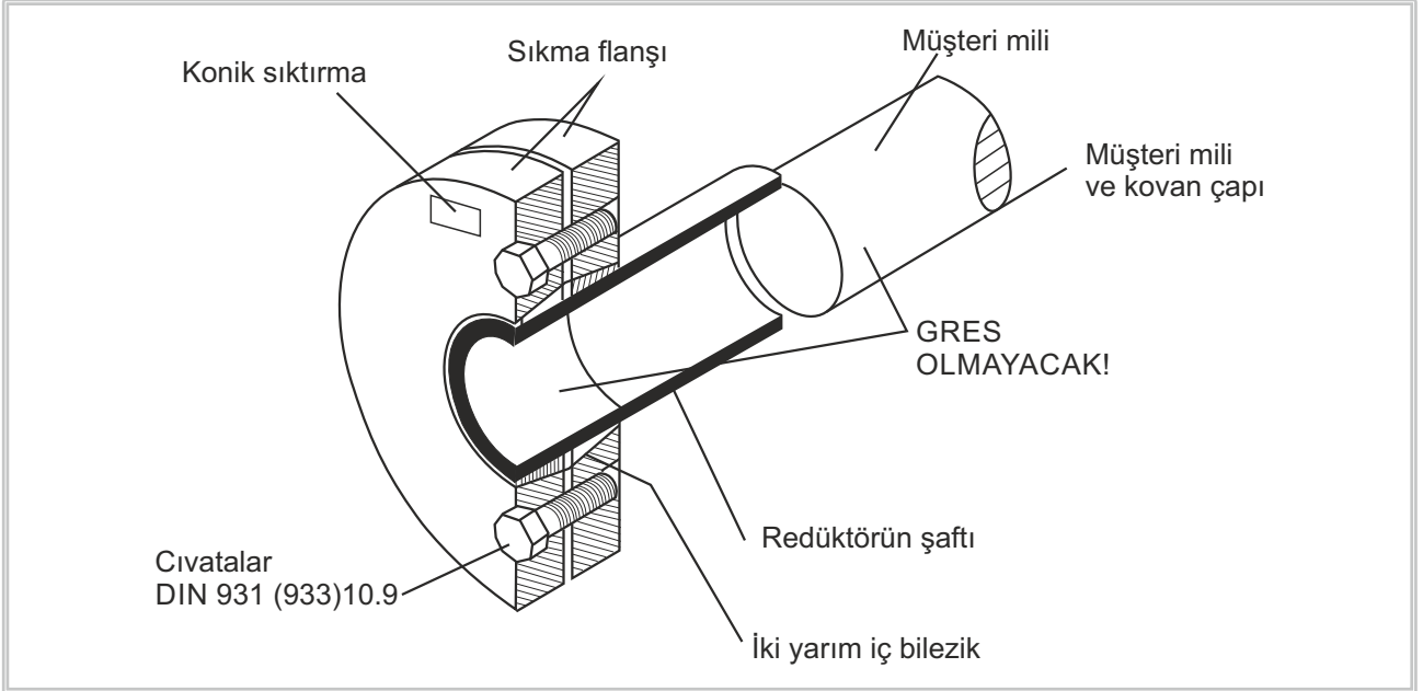
Şekil 12: Konik Sıkırma
