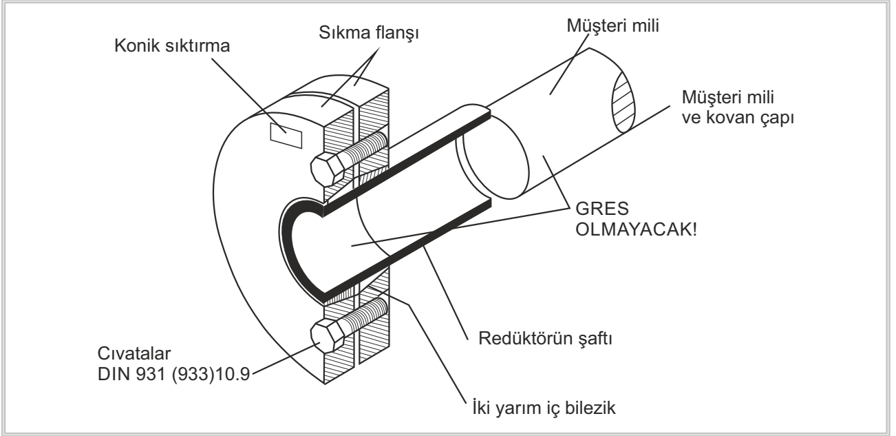
Şekil 9: Konik Sıkırma
