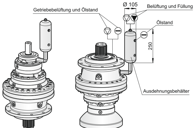
Abbildung 8: Ausdehnungsbehälter
