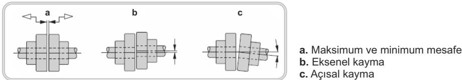
Şekil 6: Kaplin Montajı
