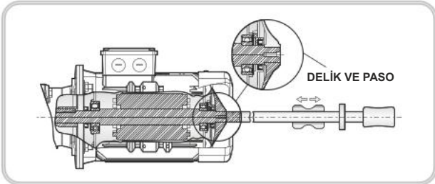
Şekil 8: Elektrik Motorunun Demontajı (PAM)
