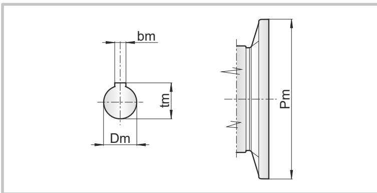
Şekil 18: PAM B14
