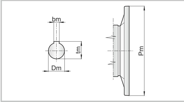
Şekil 17: PAM B5
