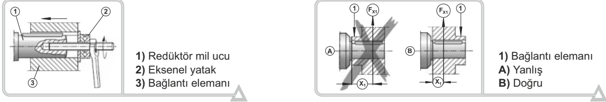
Şekil 5: Bağlantı Elemanının Çıkış Miline Montajı
