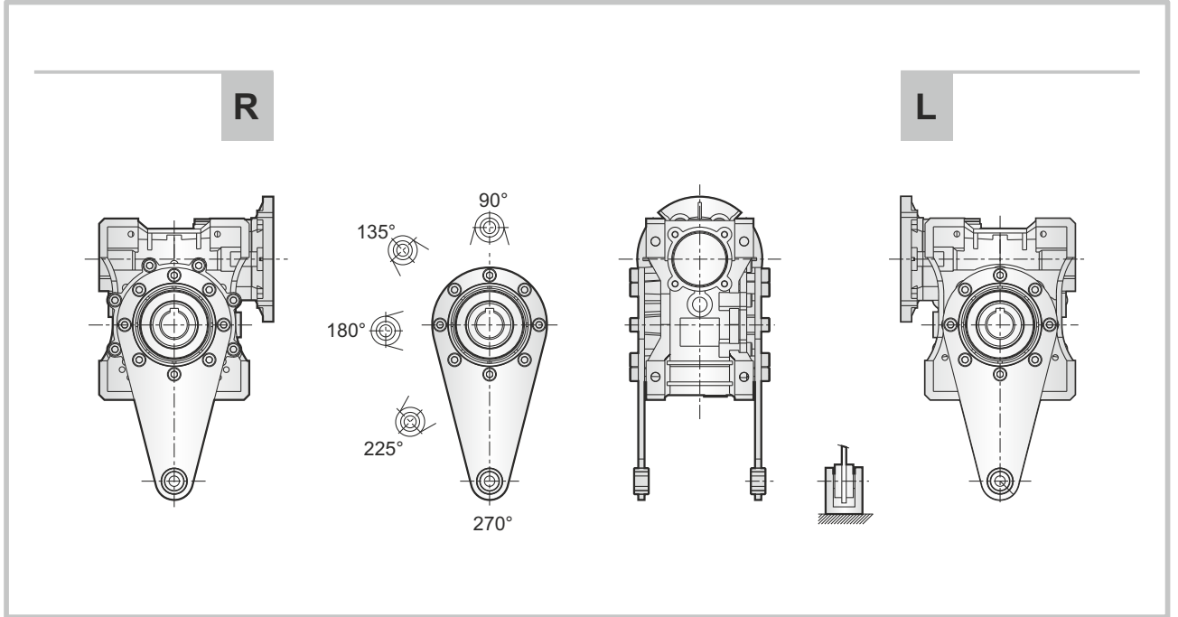
Şekil 10: Tork Kolu
