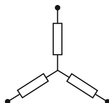
STERNAN SCHLUSS \Lambda 400 V
