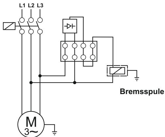
Verzögerter Bremsbetrieb (400V)
