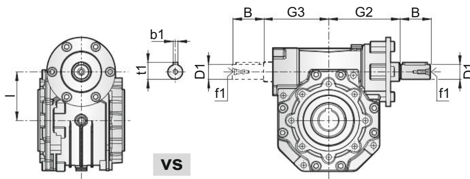
Abbildung 11: Antriebswelle (ISV)
